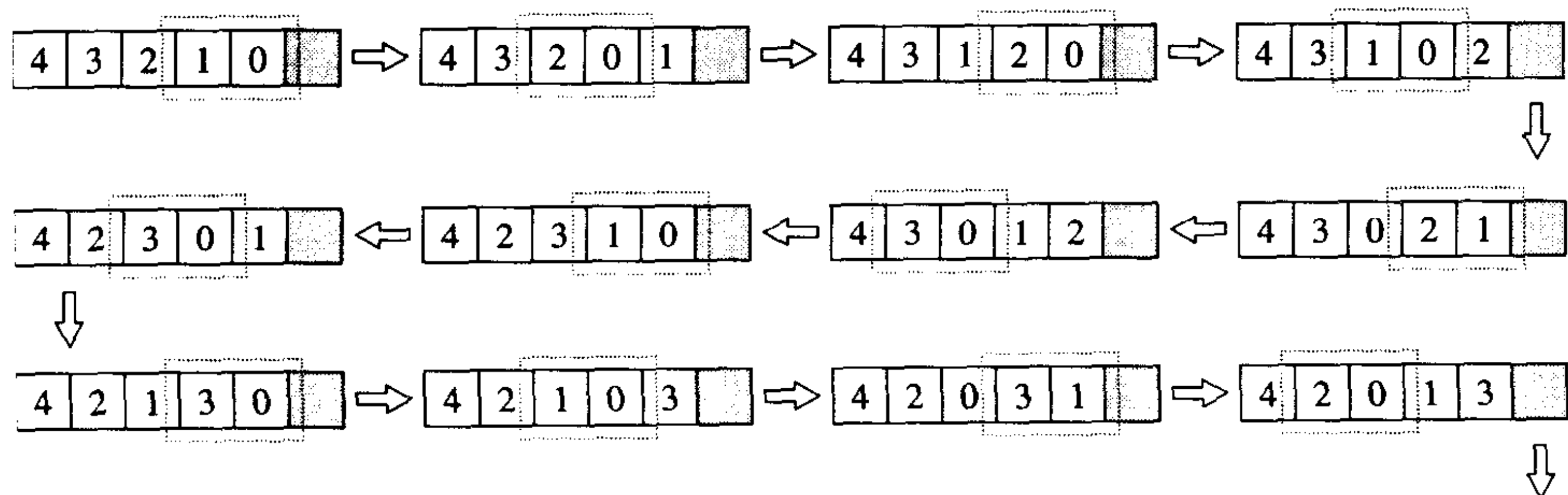
图 6-10 prev_permutation 算法 实例演练
