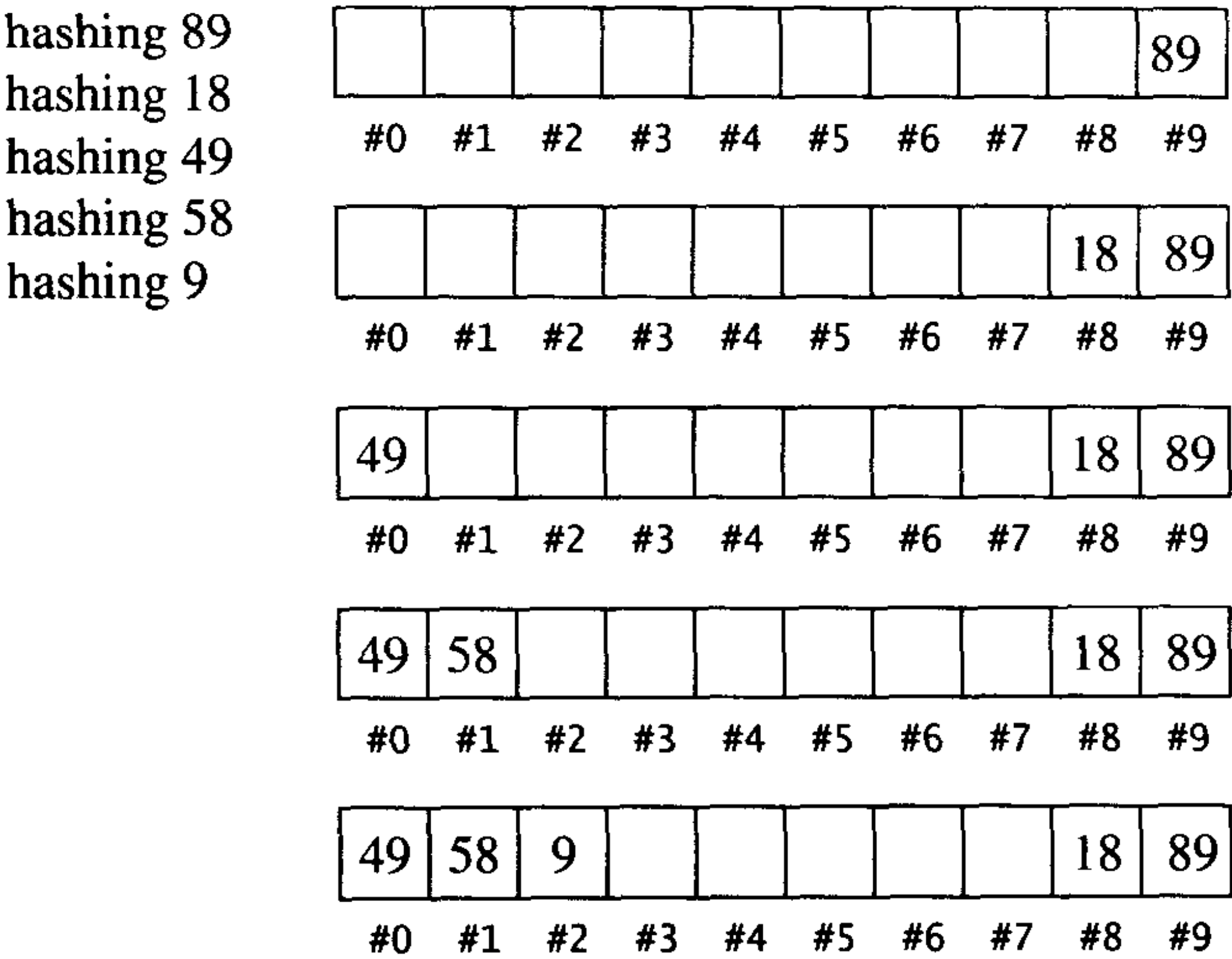
图 5-22 线性探测 (linear probing)。依序插入 5 个元素，array 的变化。
