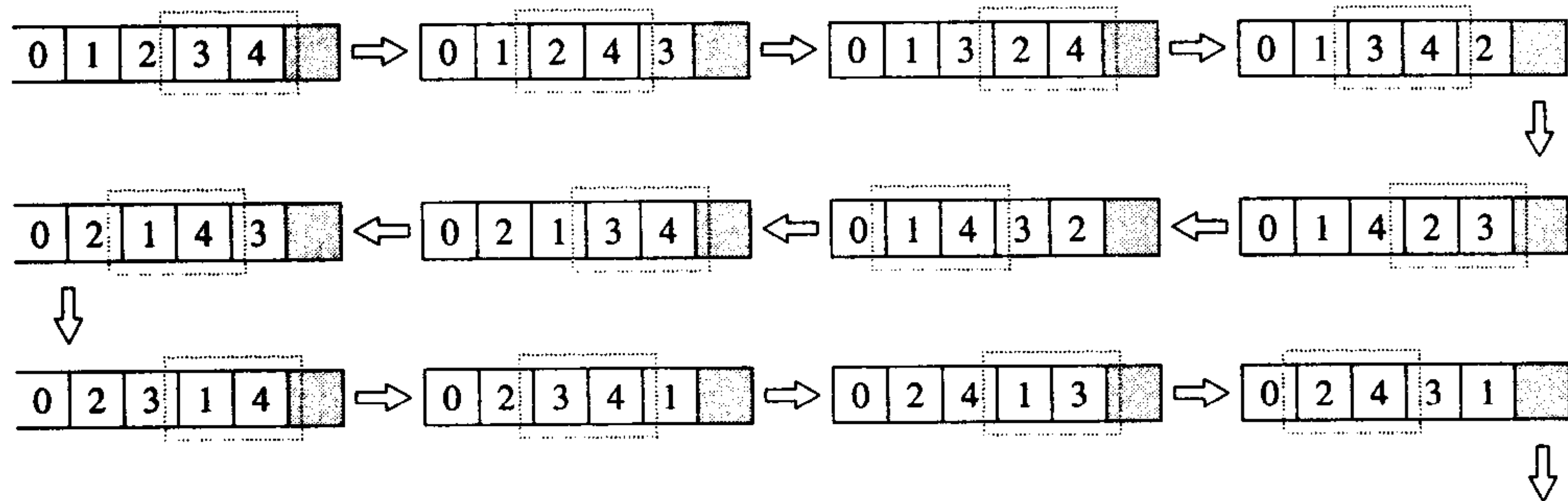
图 6-9 next_permutation 算法 实例演练
