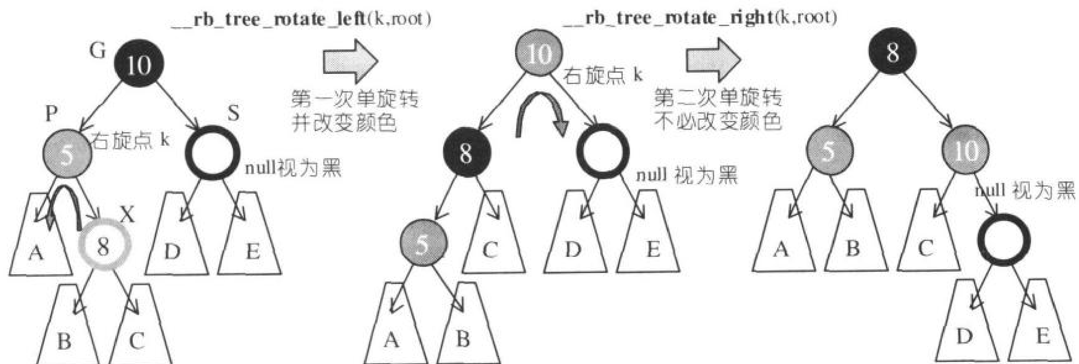
图 5-15b 最上方所示为 SGI <stl_tree.h> 所提供的函数, 用于左旋或右旋。
