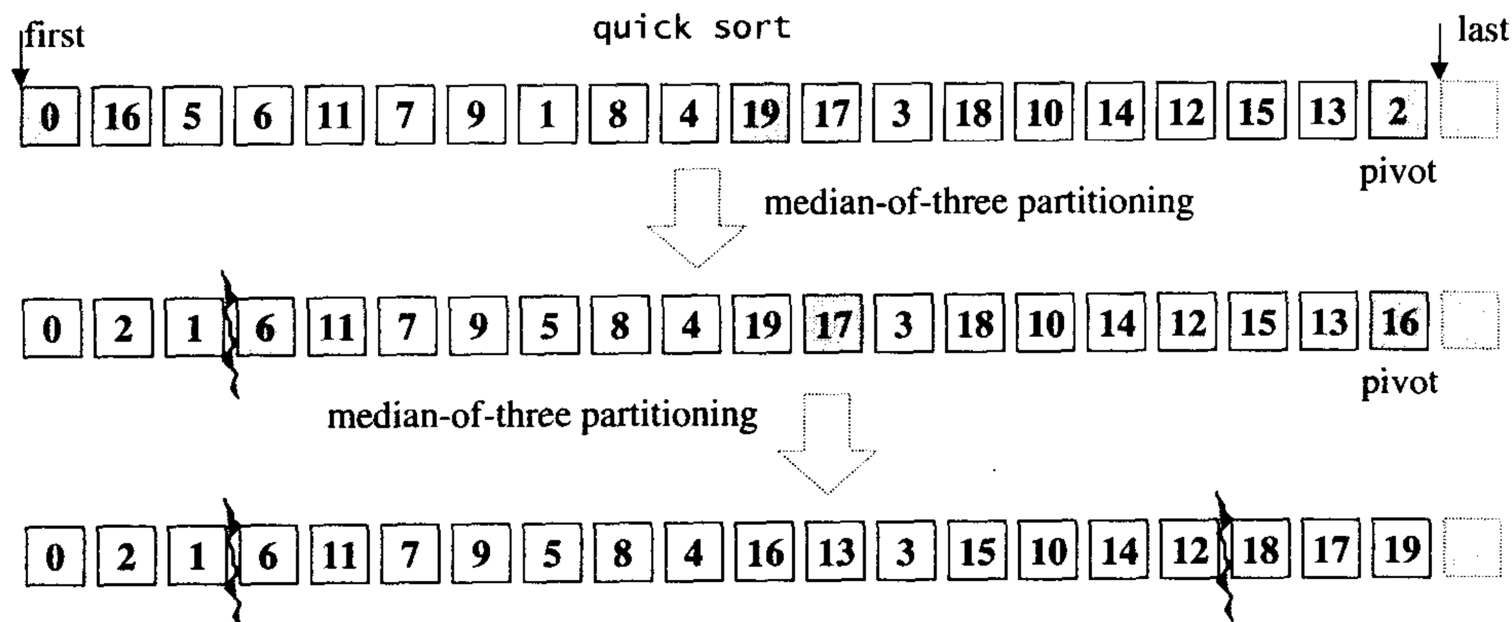
图 6-13 Quick Sort 采行分段排序。分段的原则通常采用 median-of-three (首、尾、中央的中间值)。因此，图中第一列以 2 为枢轴，分割出第二列所示的左右两段。第二列的右段再以 16 为枢轴，分割出第三列的两段。依此类推。
