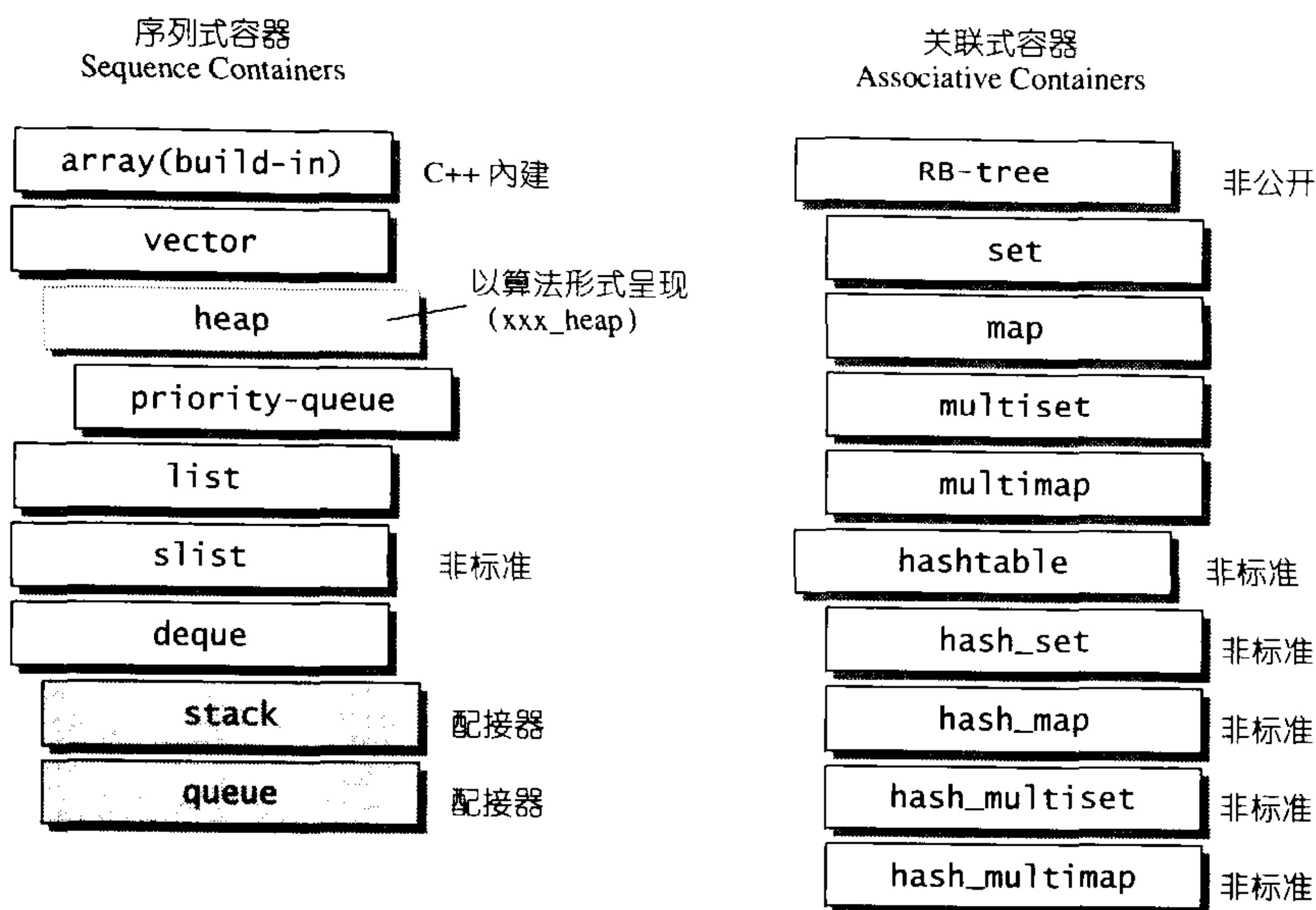
图 5-1 SGI STL 的各种容器。本图以内缩方式来表达基层与衍生层的关系。这里所谓的衍生，并非继承 (inheritance) 关系，而是内含 (containment) 关系。例如 heap 内含一个 vector, priority-queue 内含一个 heap, stack 和 queue 都内含一个 deque, set/map/multiset/multimap 都内含一个 RB-tree, hash_x 都内含一个 hashtable。
