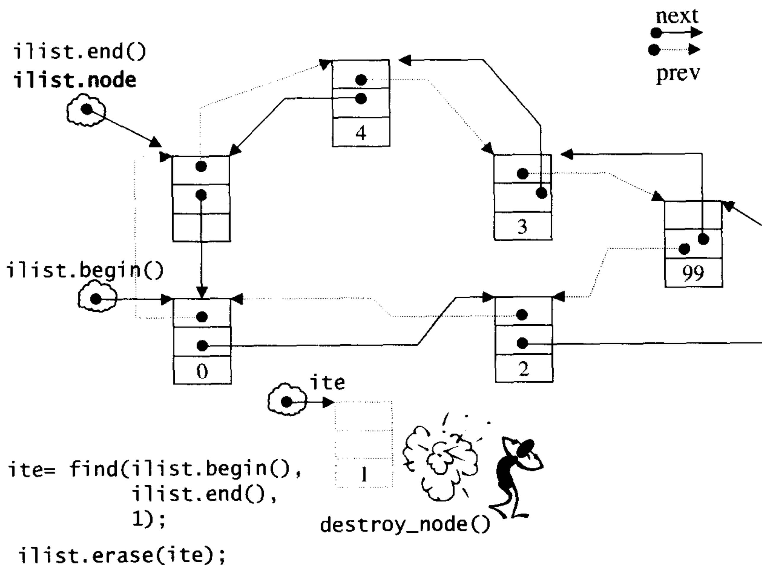
图 4-7 移除“元素值为 1”的节点
