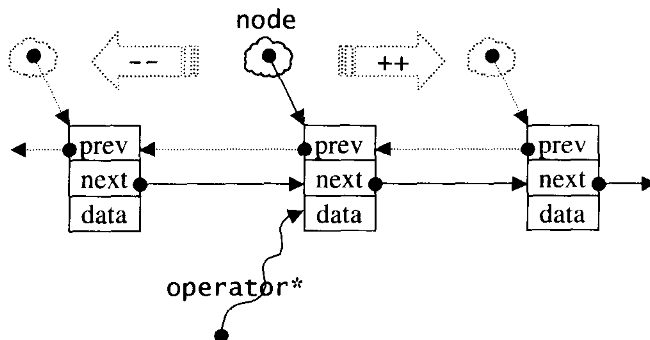
图 4-4 list 的节点与 list 的迭代器
