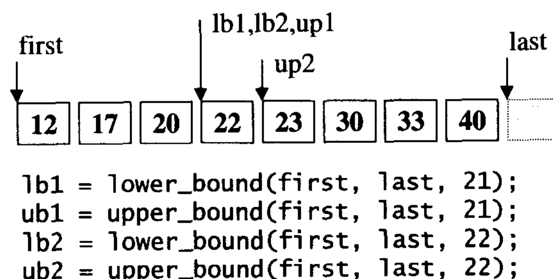
图 6-7 lower_bound 和 upper_bound
