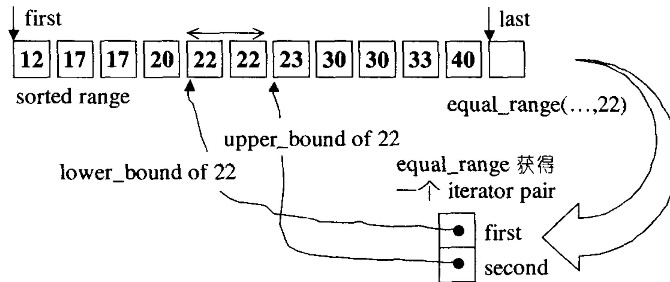
图 6-15 equal_range 的执行结果示意
