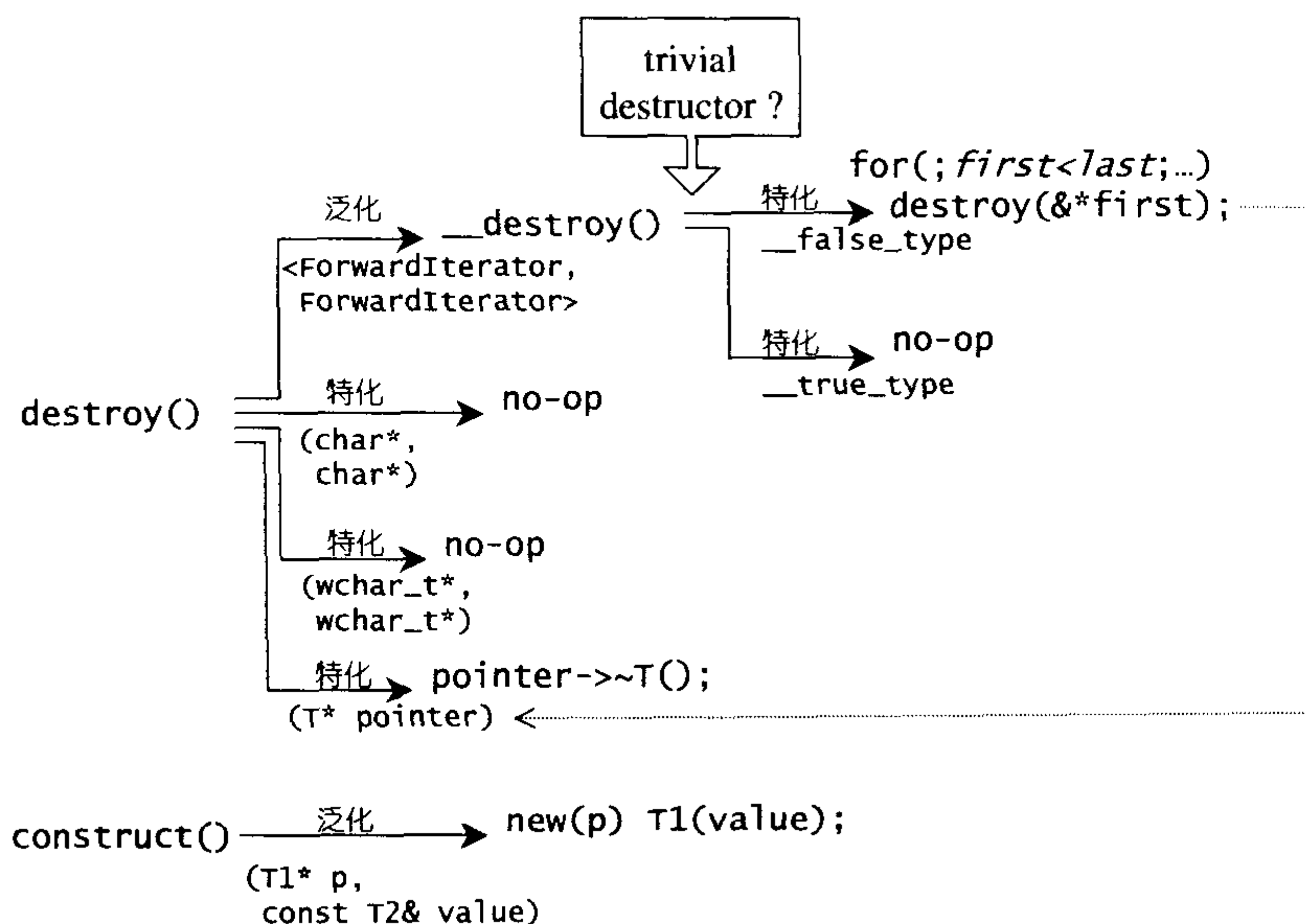
图 2-1 construct() 和 destroy() 示意
