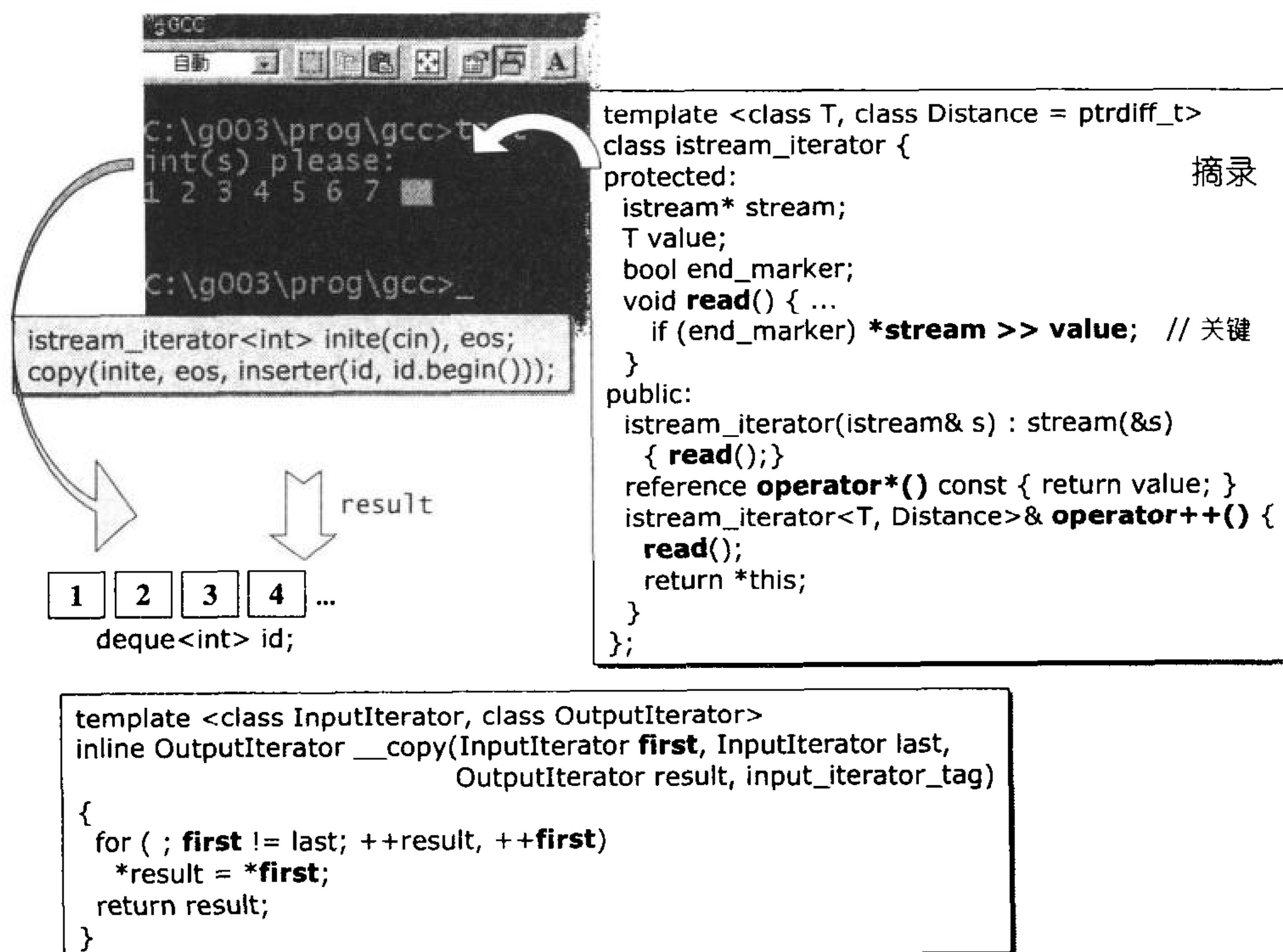
图 8-4 copy() 和 istream_iterator 合作。屏幕画面下方的浅蓝色方块是客户端程序代码, 程序流程将停在其中第一行, 等待用户从 cin 输入 (因为右侧的 istream_iterator 源代码告诉我们, 一产生 istream_iterator 对象, 便会调用 read() , 执行 *stream >> value , 而 *stream 在本例就是 cin )。用户输入数值后, copy 算法 (源代码见最下方块内容) 将该数值插入到容器之内, 然后执行 istream_iterator 的 operator++ 操作 —— 这又再次引发 istream_iterator::read() , 准备读入下一笔资料...
