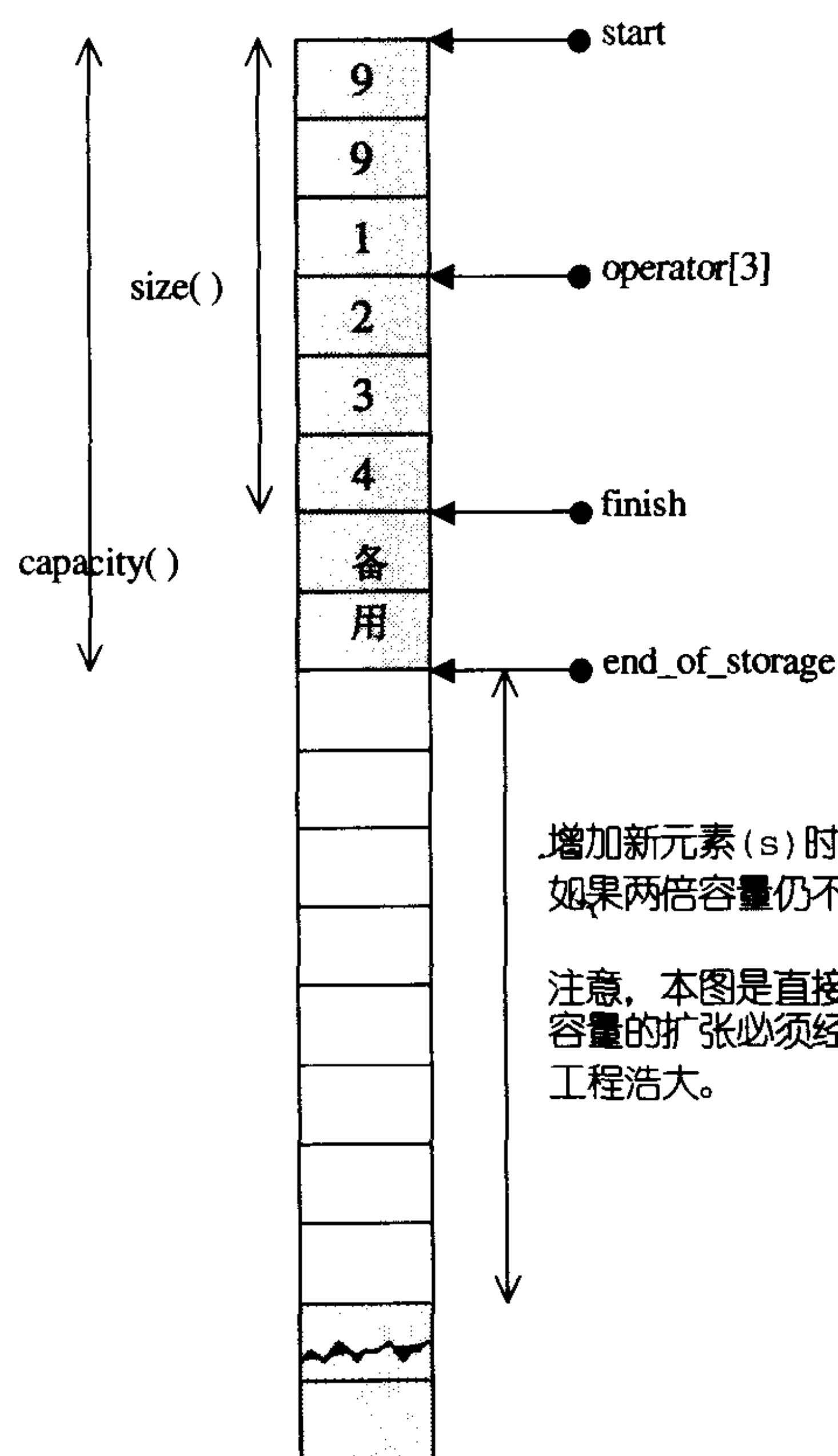
图 4-2 vector 示意图
