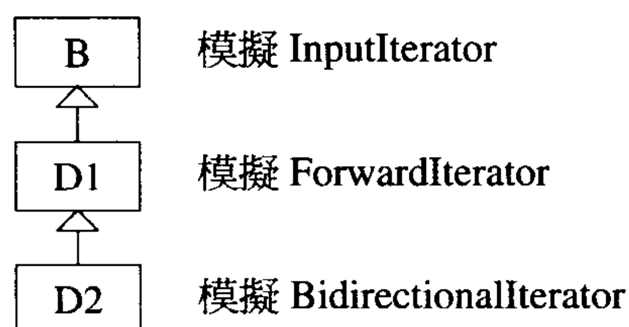
图 3-3 类继承关系
