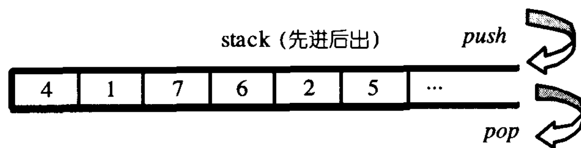
图 4-18 stack 的结构
