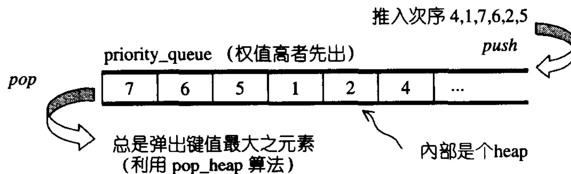
图 4-24 priority_queue
