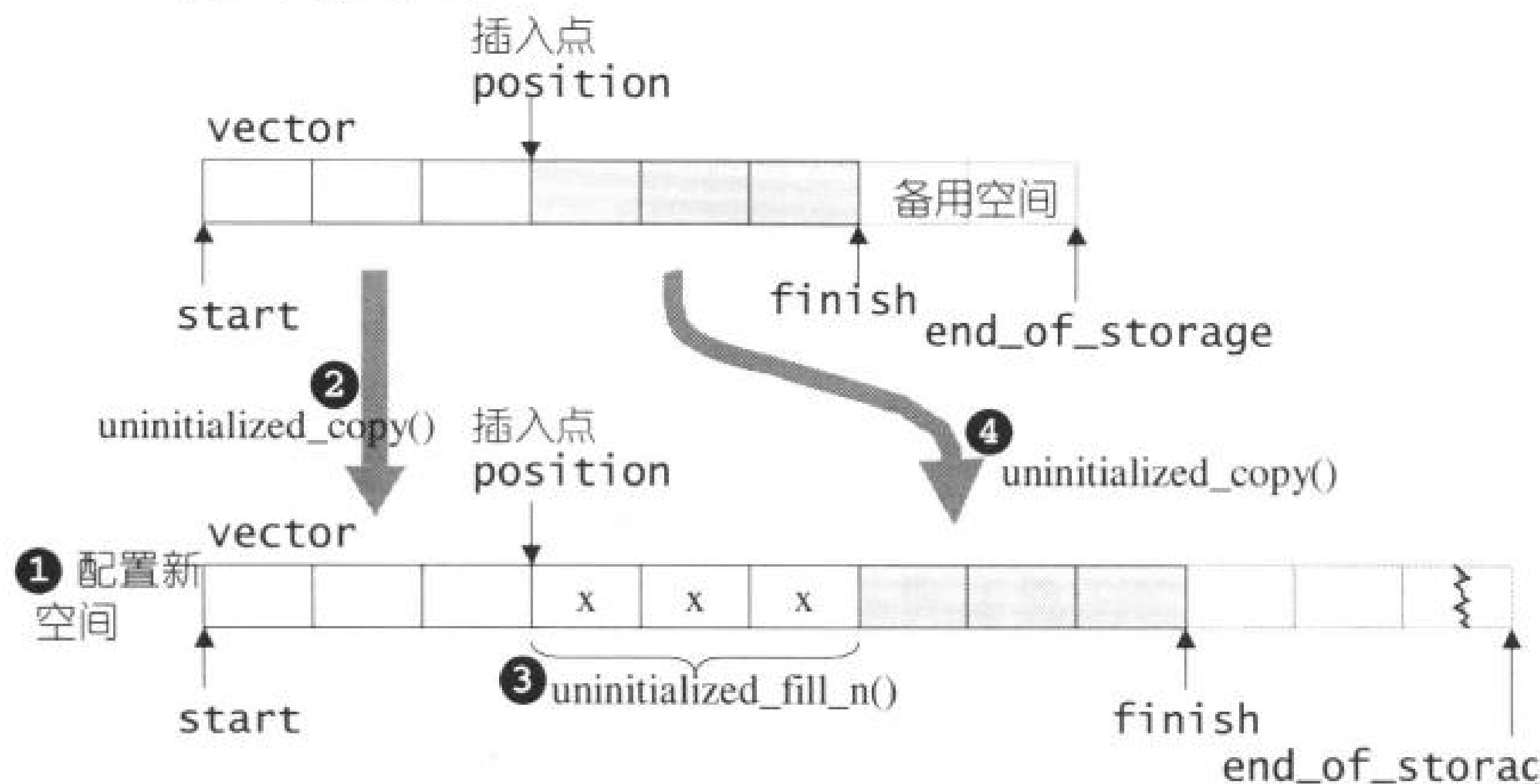
图 4-3b-3 insert(position,n,x) 状况 3
