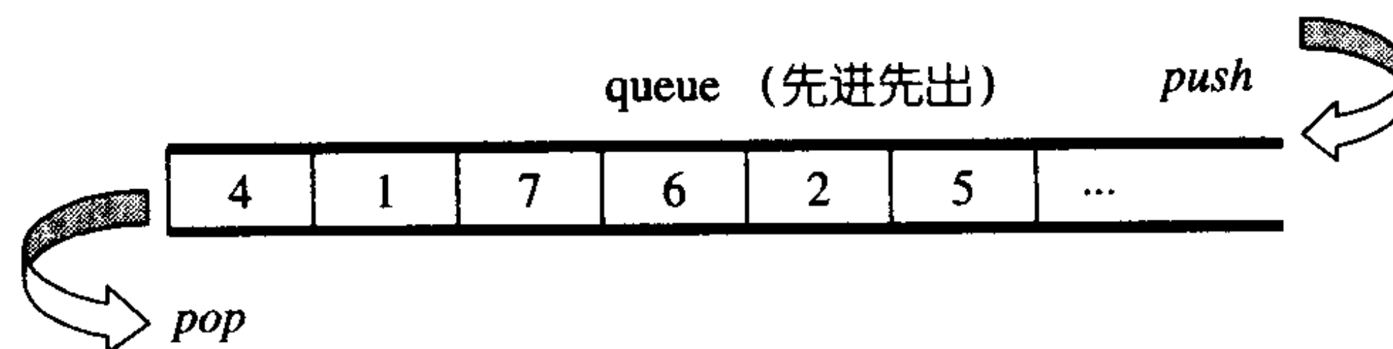
图 4-19 queue 的结构
