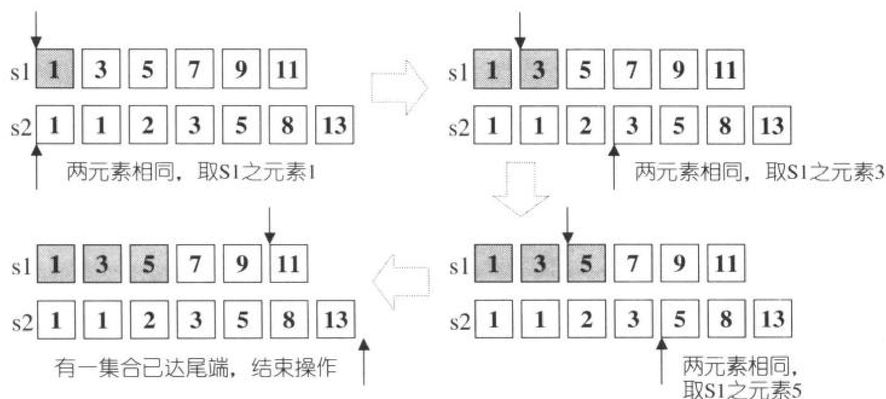
图 6-5b set_intersection 之步进分析
